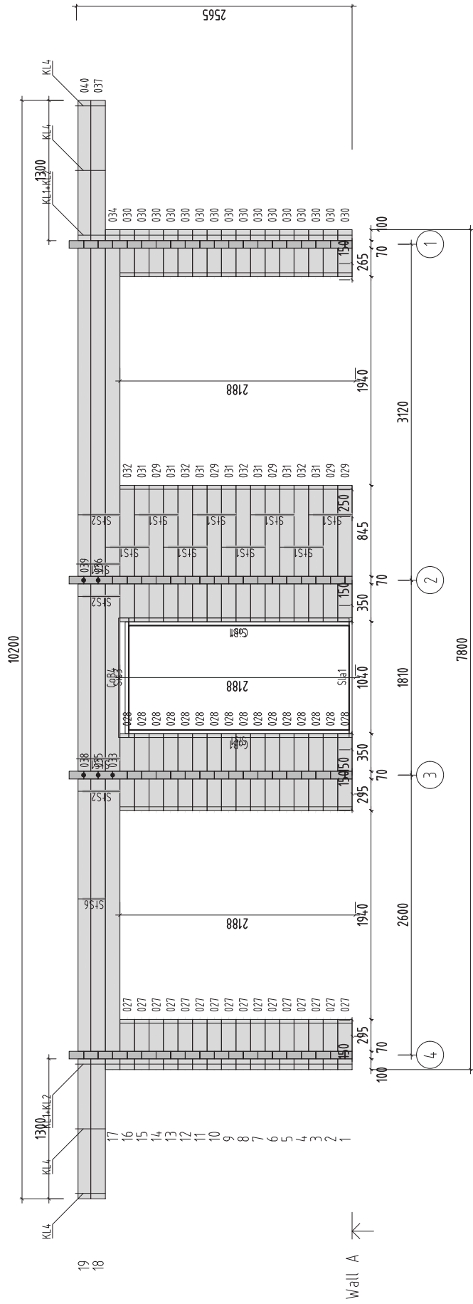
Plan 7 : WALL A plan
